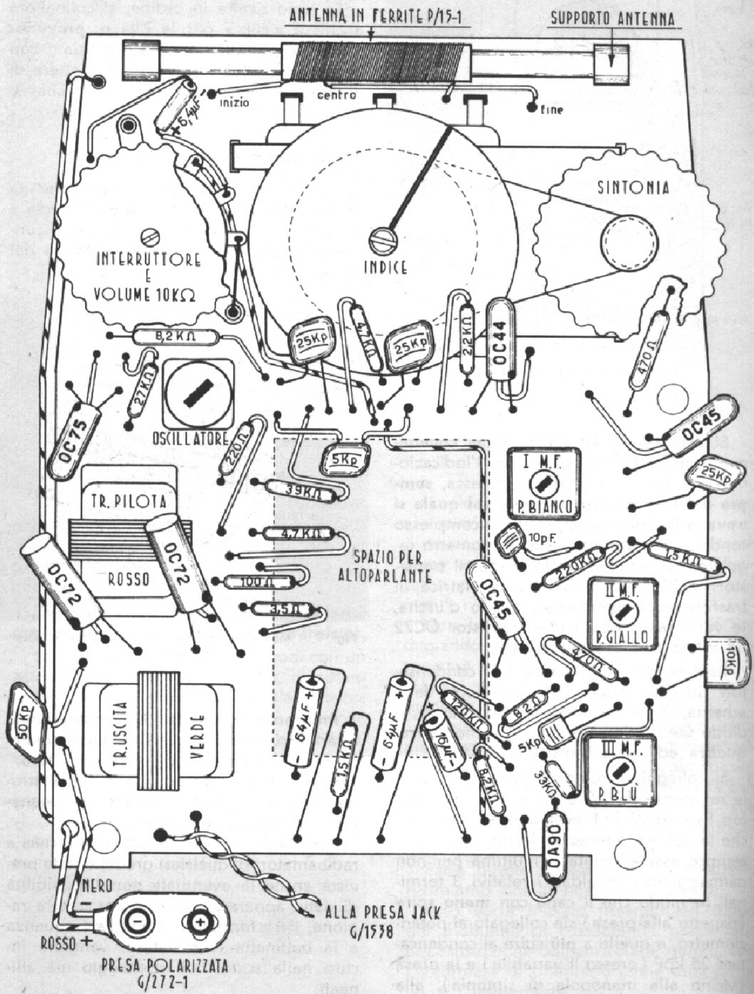
- Disposizione telaio delle connessioni stampate dei vari componenti.
